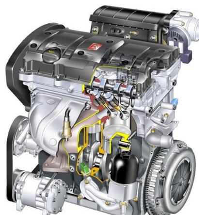
Fig. 15 Motor de combustión
