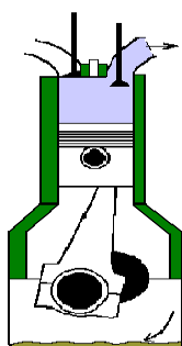
Fig. 22 Escape
