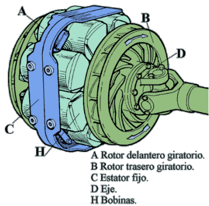
Fig. 14 Freno eléctrico
