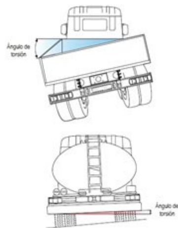
Fig. 17 Movimiento torsional
