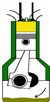
Fig. 20 Compresión
