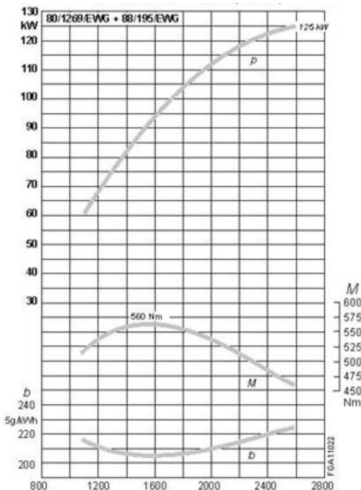
Fig. 25 Curvas de potencia, par y consumo
