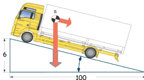
Fig. 13 Resistencia de pendiente
