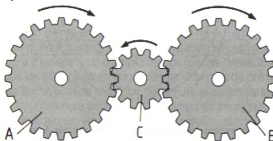
Fig. 13 Tren de engranajes
