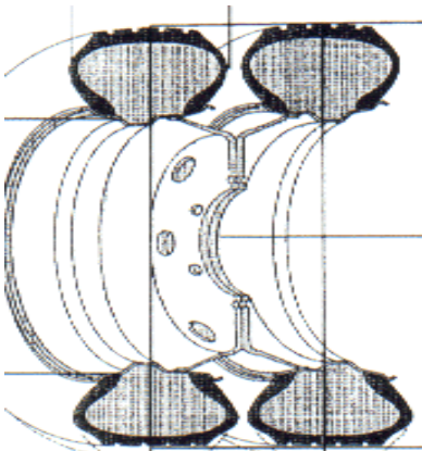
Fig. 14 Montaje gemelo
