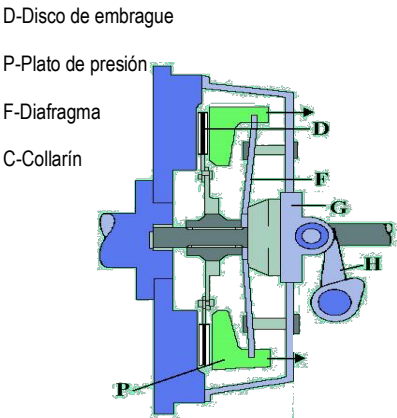
Fig. 8 Desembragado
