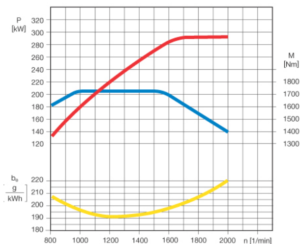
Fig. 26 Curvas características
