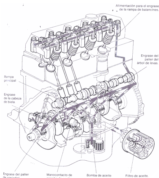
Fig. 1 Sistema de lubricación
