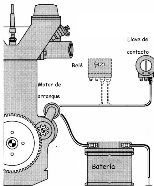
Fig. 12 Situación y conexión del motor de arranque
