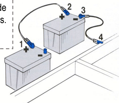
Fig. 7 Conexión de arranque con batería auxiliar
