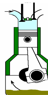
Fig. 19 Admisión
