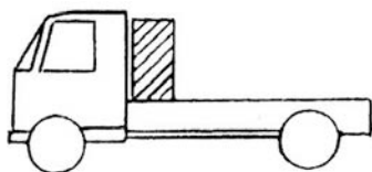
Fig. 5. Colocación incorrecta. Se puede arquear el bastidor. Sobrecarga las ruedas delanteras, produciendo un desgaste en las mismas. Agarrota la dirección.
